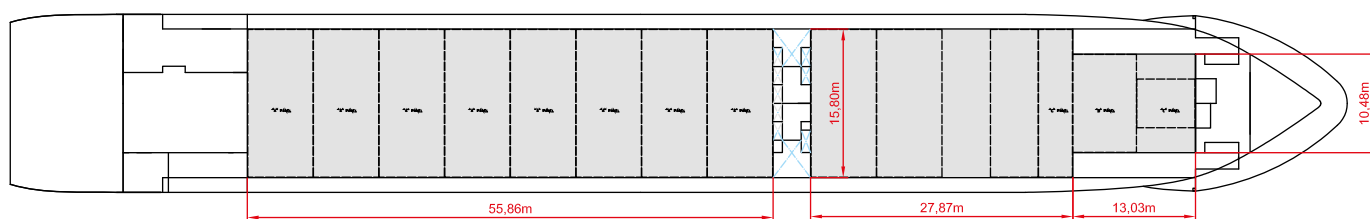
Tweendeck
